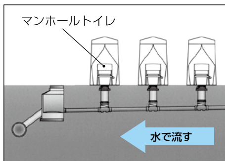
▲マンホールトイレの仕組み
