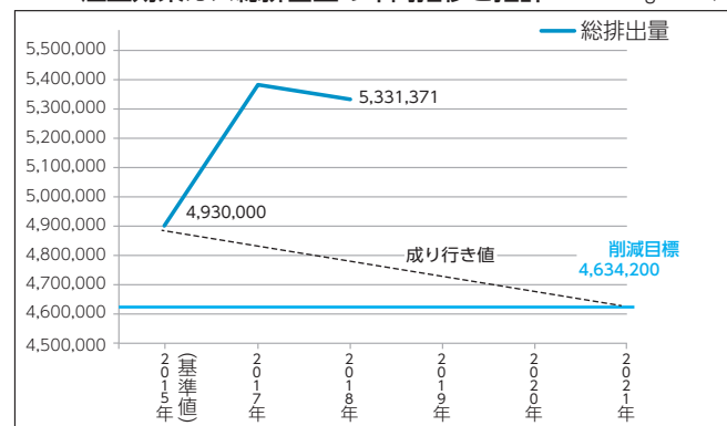
図3 温室効果ガス総排出量の年間推移と推計（単位：kg/CO 2 ）
