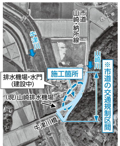
【①山崎川河道切替工事】
