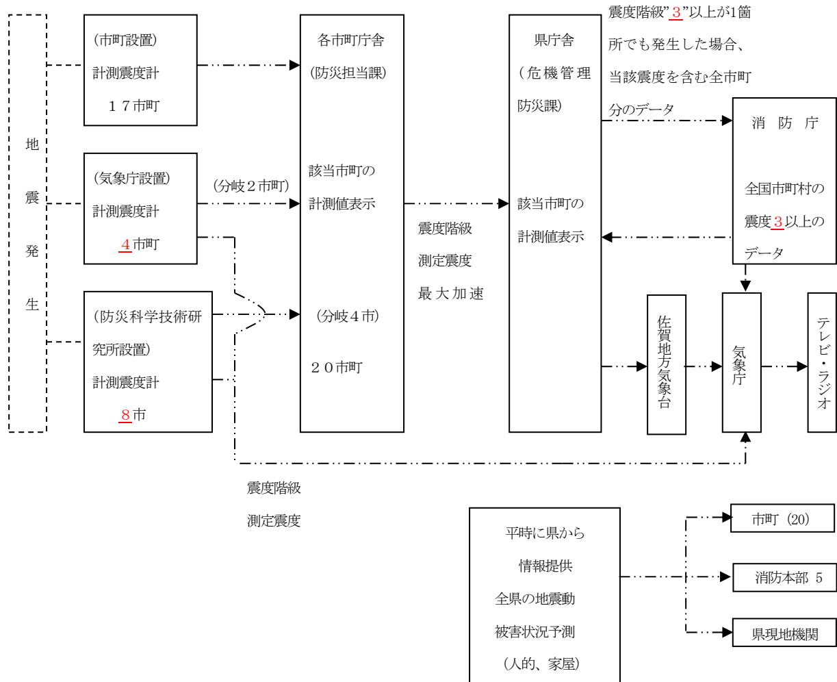
【佐賀県震度情報ネットワークシステム図】
