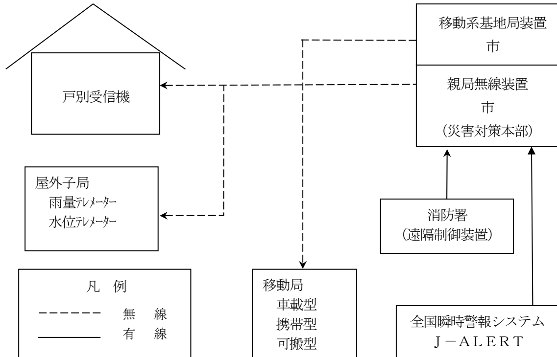
【市防災行政無線系統図】
